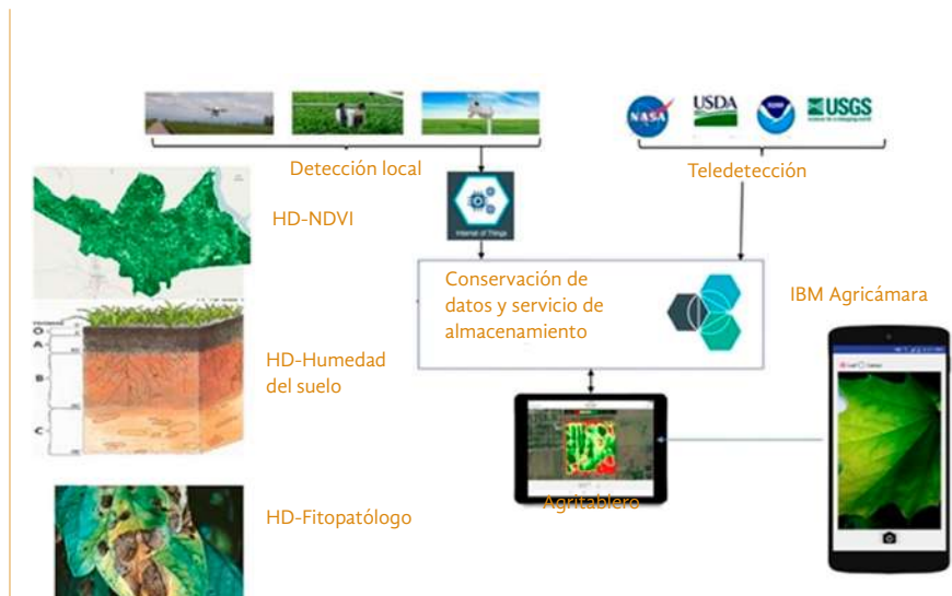
Figura 1. Integración de teledetección utilizando el IoT y servicios de computación en la nube en la agricultura de precisión (adaptado de IBM, 2018).
