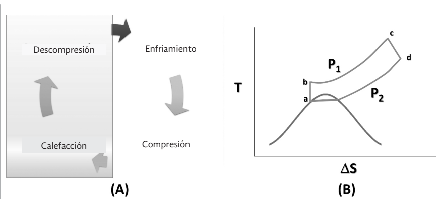
Figura 2. Ciclo de Brayton para el procesamiento eficiente del dióxido de carbono supercrítico. (A) Esquema de los diversos pasos del ciclo de Brayton. (B) Esquema de un diagrama de temperatura - entropía del ciclo de Brayton: (a -> b) compresión isentrópica (o adiabática), (b -> c) calentamiento isobárico en P_1 , (c -> d) descompresión, (d -> a) enfriamiento isobárico, hasta llegar a las condiciones subcríticas en P_2 .
