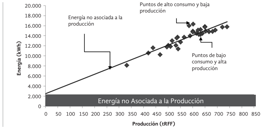
Figura 3. Tendencia de consumo vs. producción para planta de beneficio.
