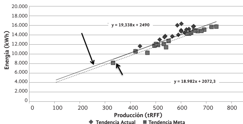
Figura 5. Comportamiento consumo de energía vs. producción – PB.
