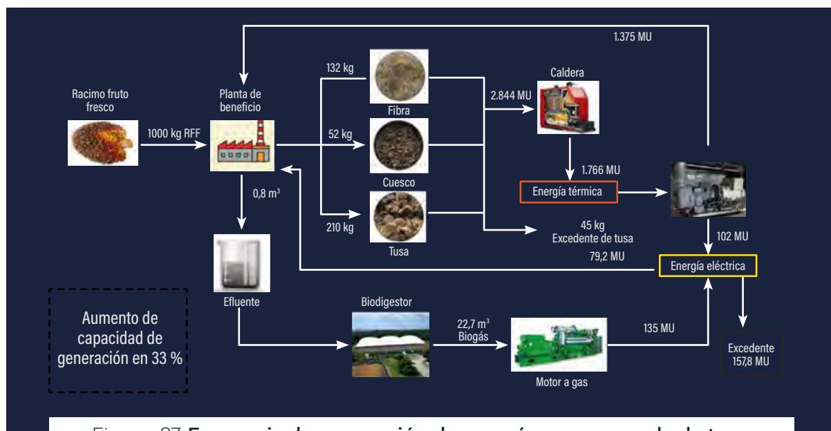
Figura 27. Escenario de generación de energía con quemado de tusa
